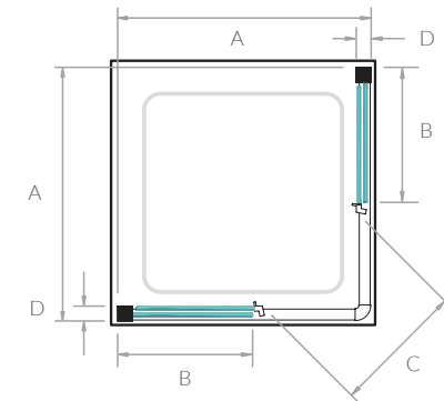
Straight Sliding Door
