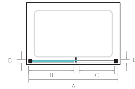
Straight Sliding Door
