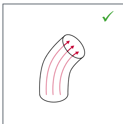
45° bend. Advisable.
